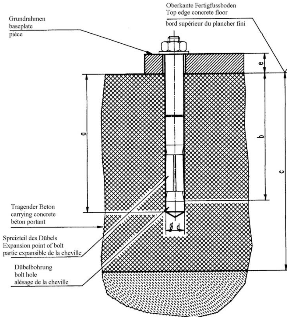
Bild 6: Auswahl der Dübellänge (ohne Bodenbelag)
