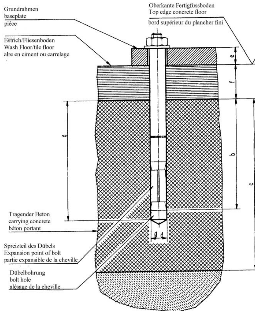
Bild 7: Auswahl der Dübellänge (mit Bodenbelag)
