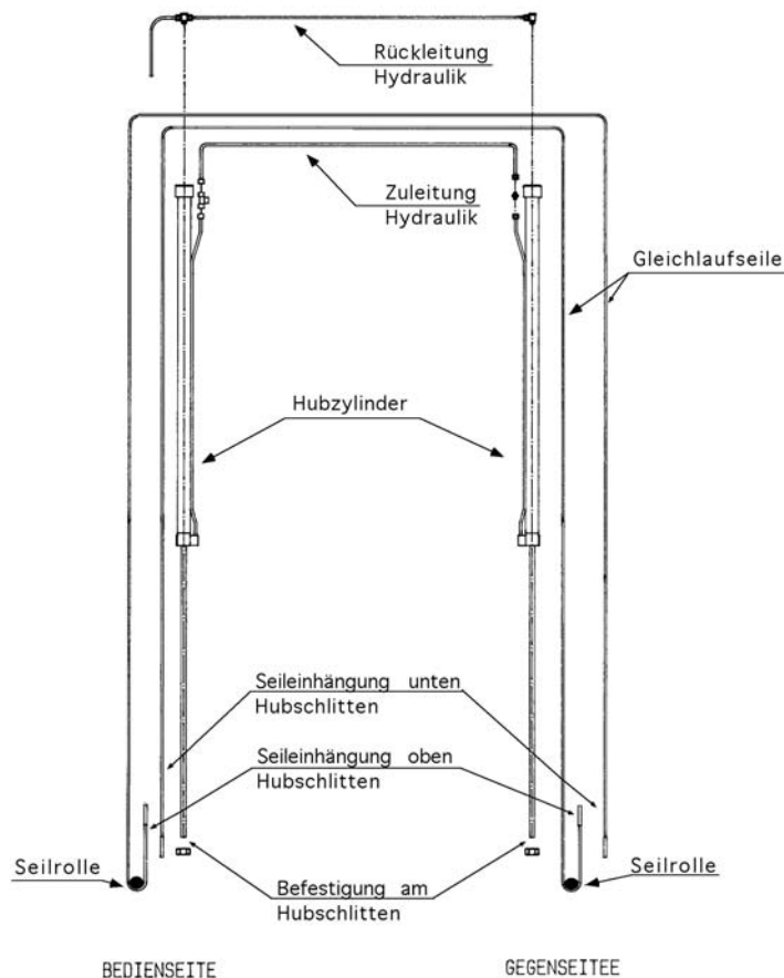
Bild 5: Seilverlauf und Hydraulikleitungen
