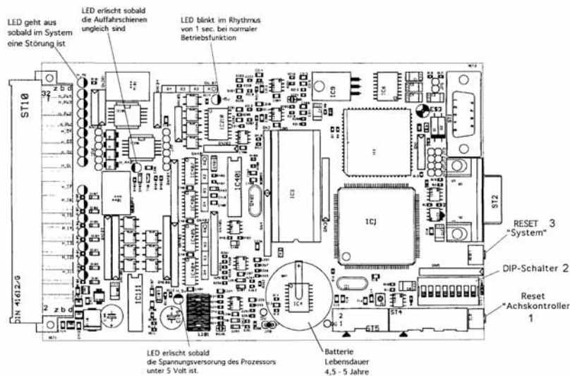
Bild 4: Achskontroller
