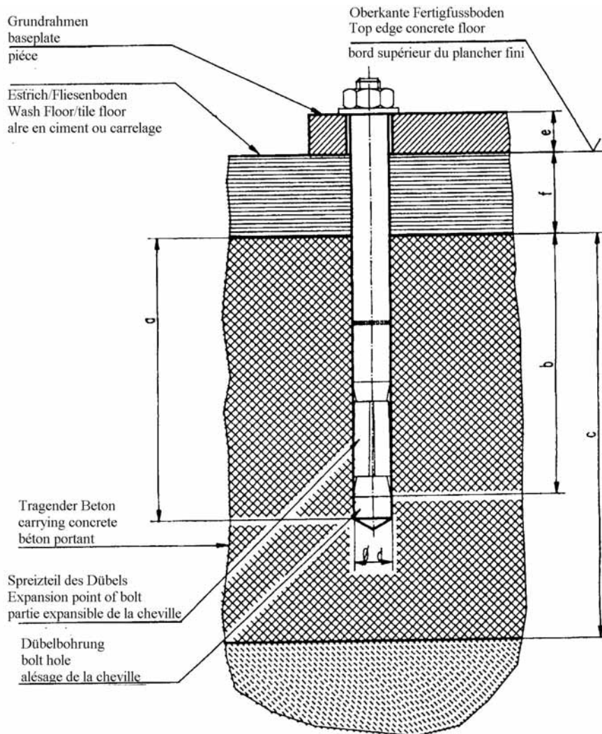
Bild 7: Auswahl der Liebig-Dübel mit Bodenbelag (Estrich, Fliesen)
