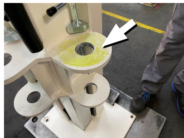
Ingrassare il braccio portante con un grasso multiuso privo di acidi
