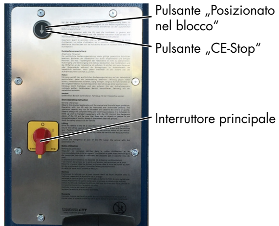
Immagine 4: Unità di comando
