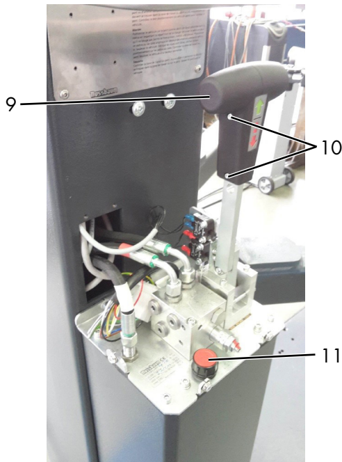
9 Bedienhebel
