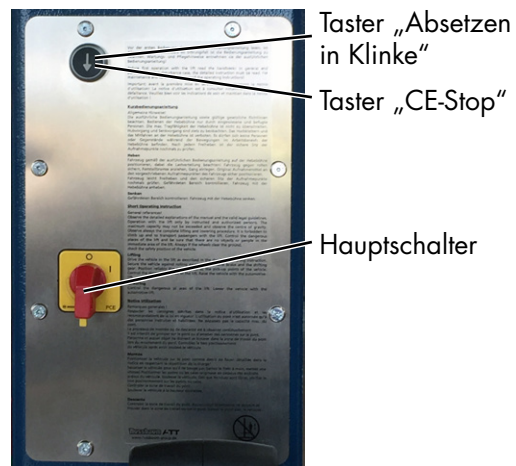
Bild 4: Bedieneinheit
