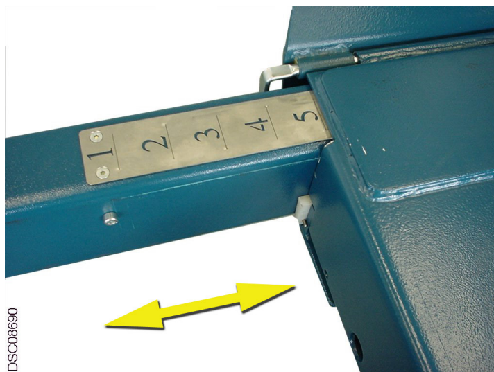
Verstellbare Auffahrschiene
