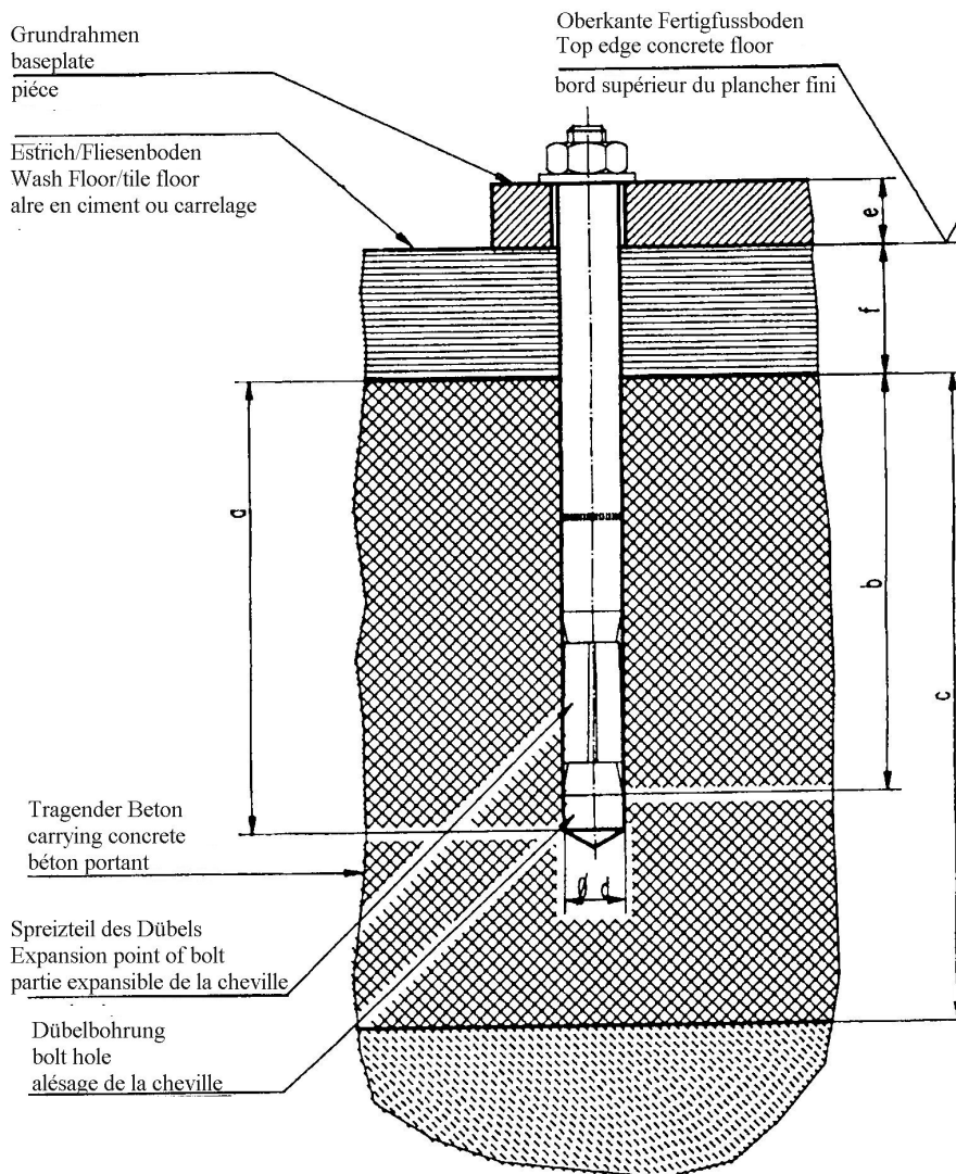
Bild 10: Auswahl der Liebig-Dübel mit Bodenbelag (Estrich, Fliesen)
