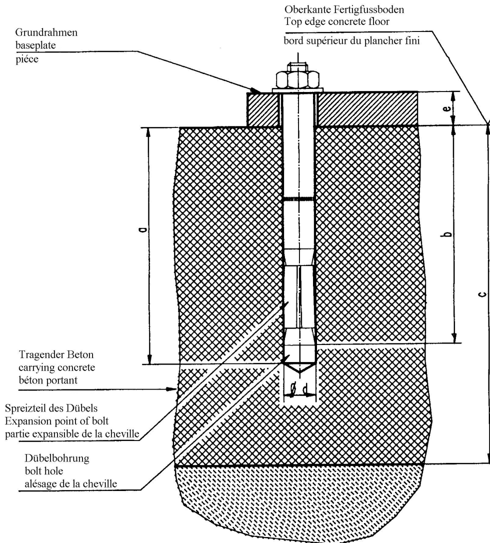
Bild 9: Auswahl der Dübellängen (ohne Bodenbelag)
